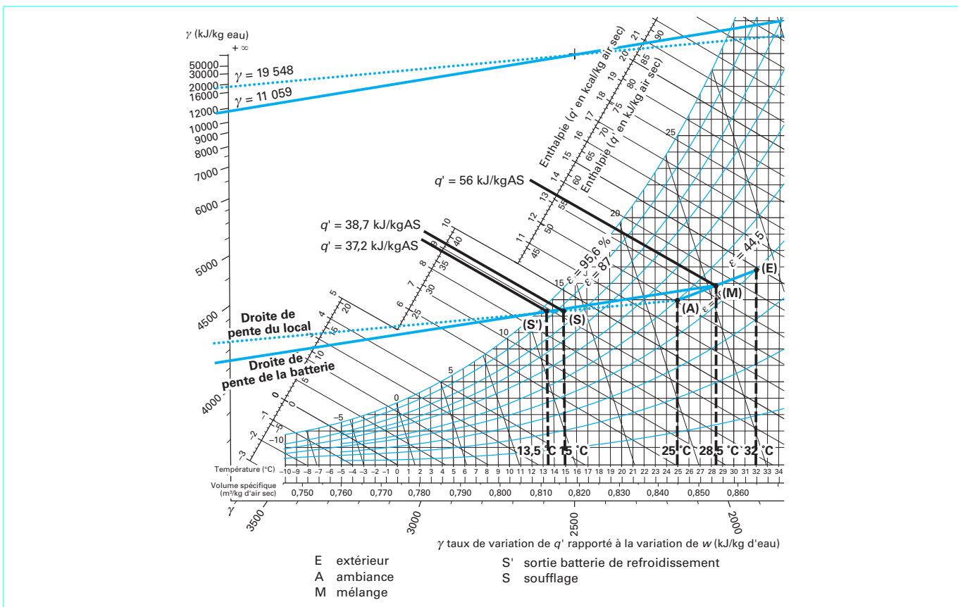
Figure 19 – Évolution de l'air dans une batterie de refroidissement et déshumidification, cas du laboratoire industriel
