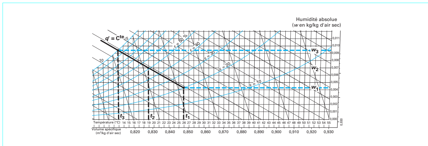
Figure 20 – Évolution de l'air dans un humidificateur adiabatique
