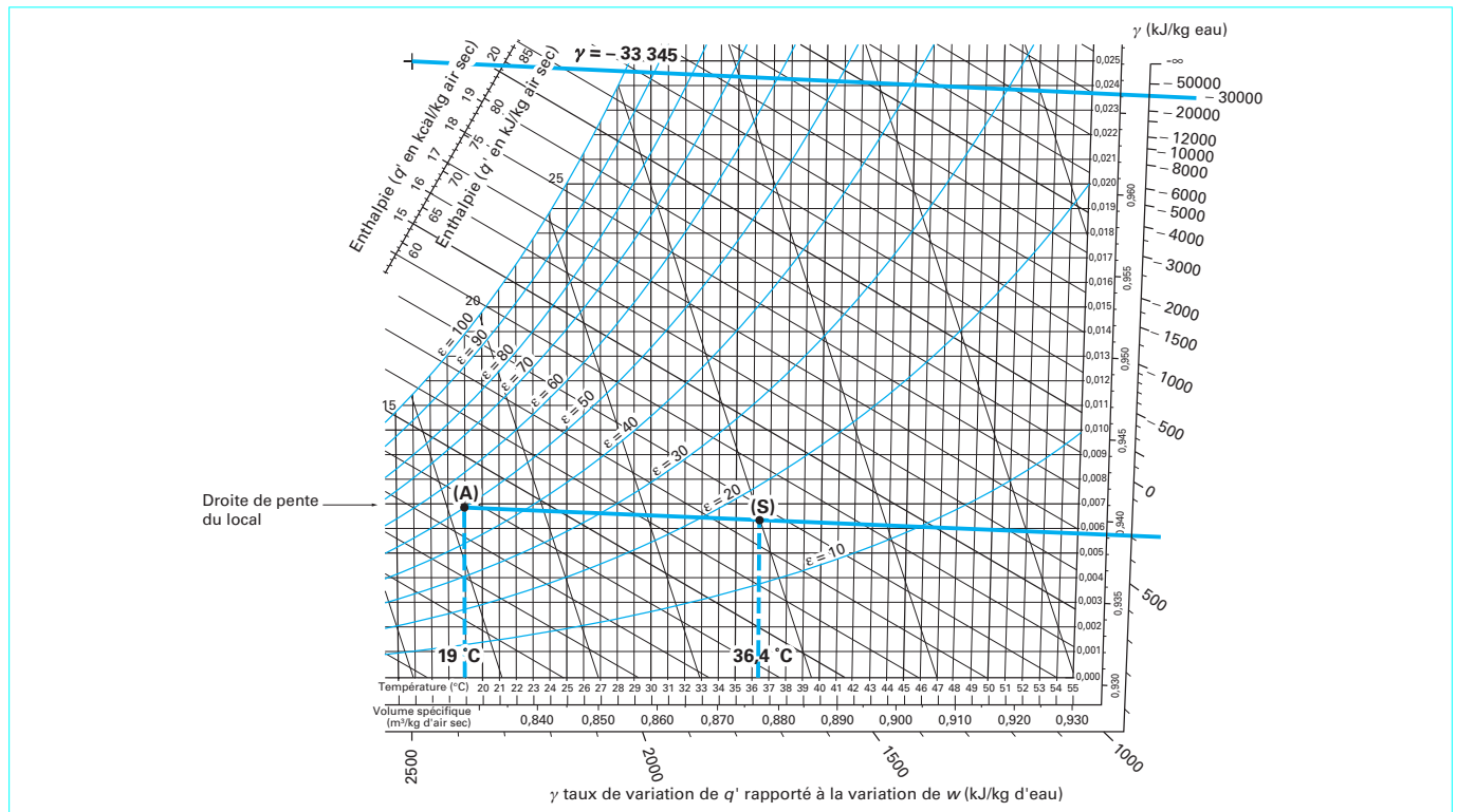
Figure 4 – Droite de pente du local en hiver hors occupation
