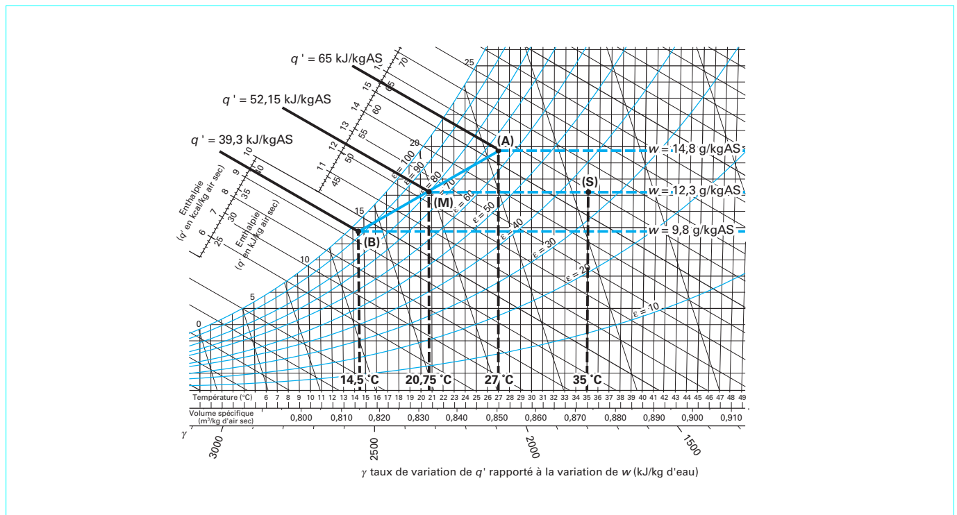
Figure 11 – Évolution de l'air avec bypass
