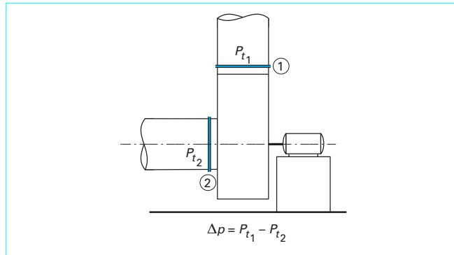
Figure 24 – Emplacement des mesures pour obtenir la différence de pression totale d'un ventilateur
