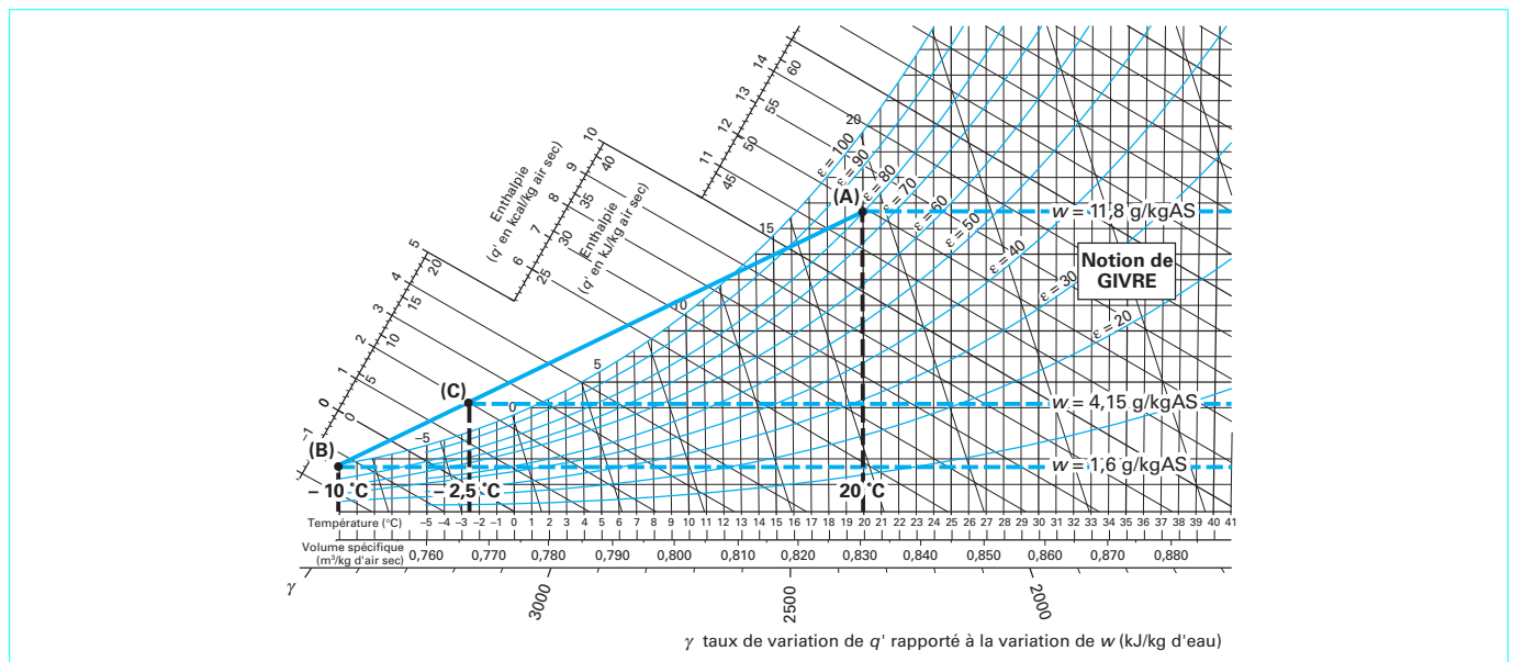
Figure 7 – Mélange en zone de givre
