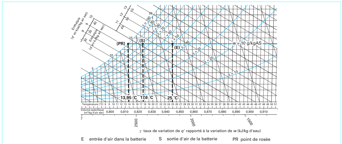
Figure 13 - Refroidissement sans déshumidification
